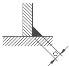
Kehlnaht A - Schuh
